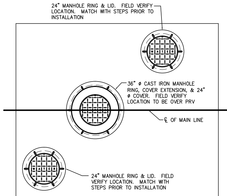
TOP VIEW LID
